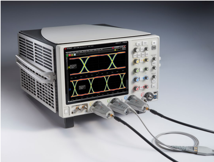
Входные тракты с малым шумом осциллографов Infiniium серии V и революционный адаптер активной нагрузки обеспечивают наилучшую в отрасли целостность сигналов.
