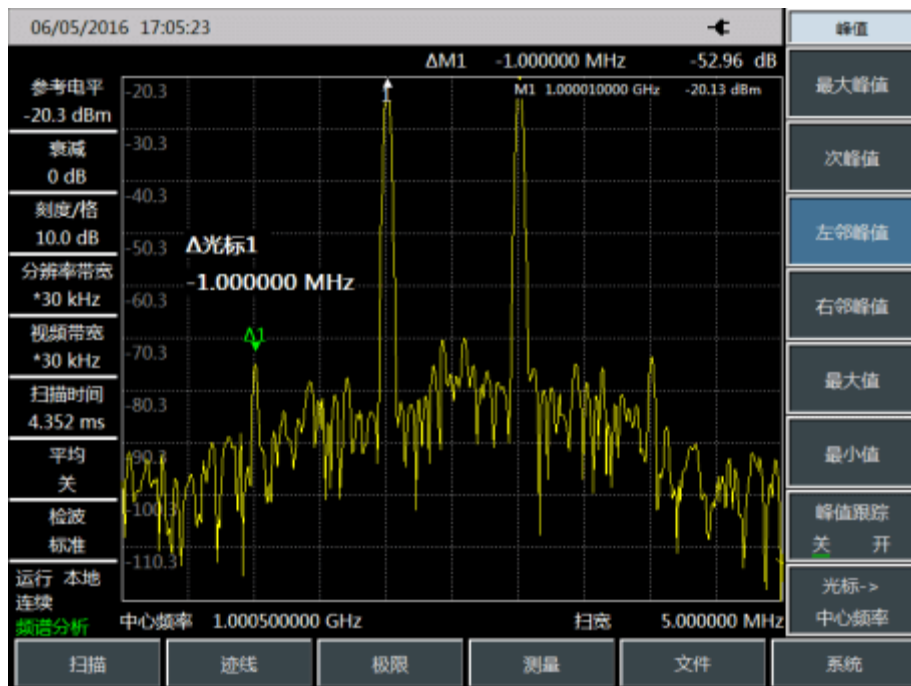
Рис.4 Относительное измерение искажений внутренней модуляции
