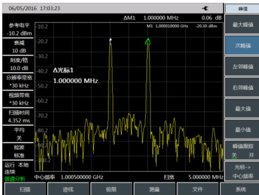
Рис. 2 Сигналы в центре дисплея анализатора спектра
