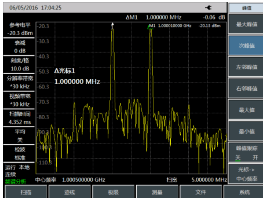
Рис. 3 Пик сигнала на опорный уровень
