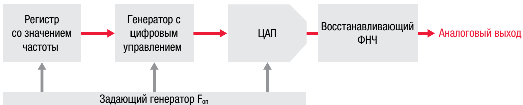
Рисунок 8. Функциональная блок-схема синтезатора на основе прямого цифрового синтеза.
