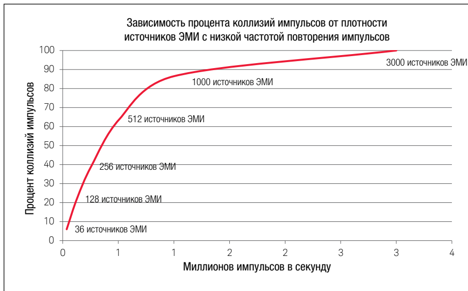
Рисунок 2. По мере роста числа источников ЭМИ растет и число коллизий импульсов, даже если все эмиттеры работают с низкой плотностью импульсов.
