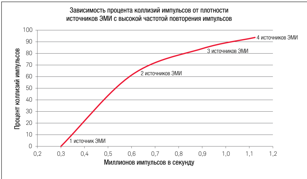
Рисунок 3. При включении в модель источников ЭМИ с высокой частотой повторения импульсов процент коллизий импульсов резко возрастает.
