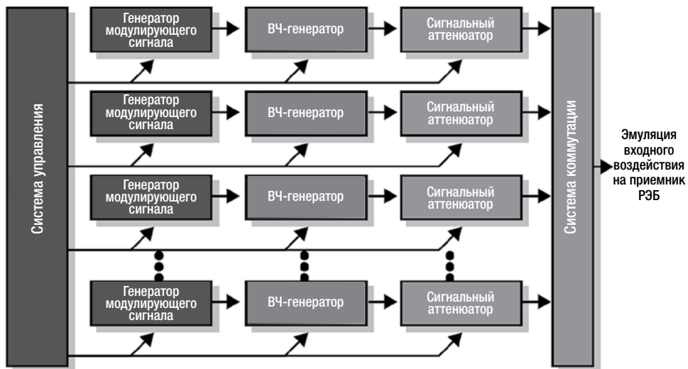
Рисунок 7. Подход к формированию сигналов с использованием отдельных функциональных элементов позволяет просто увеличивать масштаб системы для повышения плотности импульсов и создания более реалистичной сигнально-помеховой обстановки. К сожалению, с ростом масштаба системы также растет ее стоимость и размер. 1
