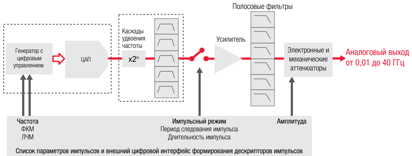
Рисунок 10. Высокоуровневая функциональная блок-схема генератора сигналов с быстрой перестройкой частоты на основе прямого цифрового синтеза, работающего в диапазоне от 0,01 до 40 ГГц.
