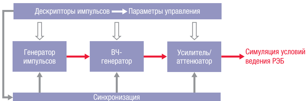
Рисунок 6. При использовании традиционного подхода для формирования и изменения требуемого сигнала параметры управления в виде дескрипторов импульсов посылаются параллельно на несколько функциональных элементов для каждого импульса. Такой подход приводит к созданию сложных систем, требующих точной синхронизации.
