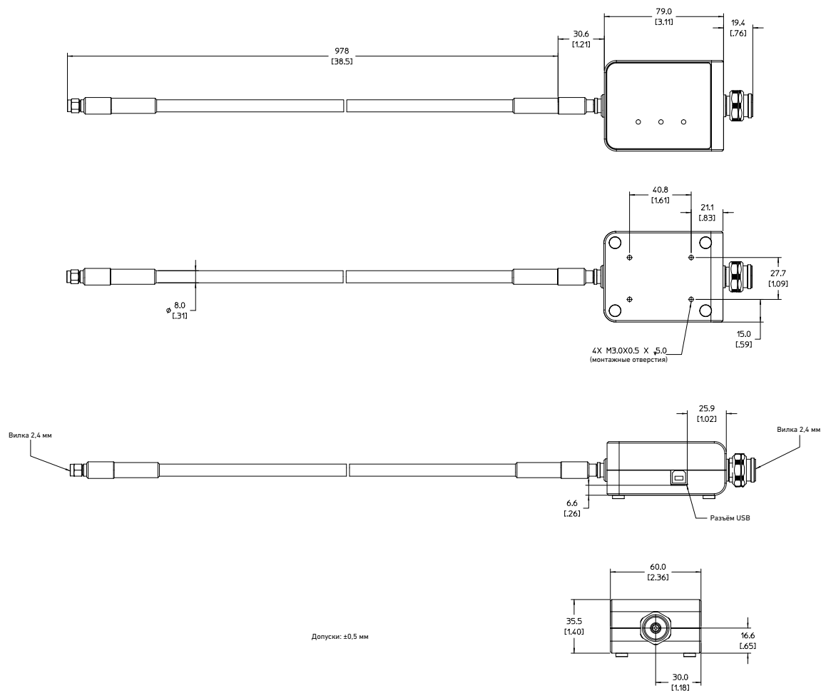
Рисунок 3-23 Размеры U7227F
