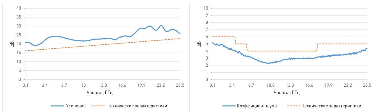
Рисунок 3-8 Keysight U7227C, зависимость усиления от частоты (типová)
