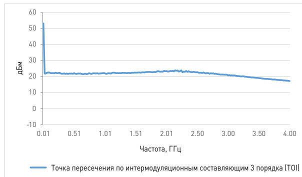
Рисунок 3-7 Keysight U7227A, зависимость точки пересечения по интермодуляционным составляющим 3 порядка (TOI) от частоты (типичная)
