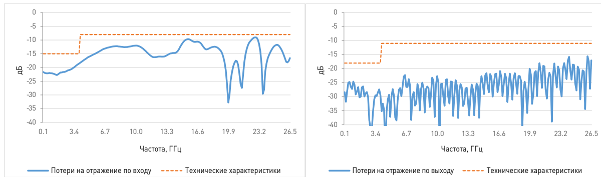
Рисунок 3-10 Keysight U7227C, зависимость потерь на отражение по входу от частоты (типová)
