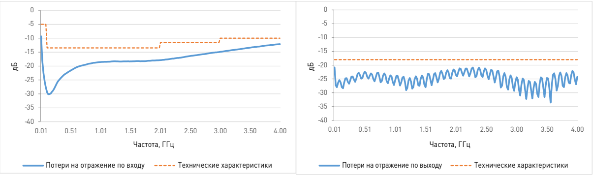
Рисунок 3-3 Keysight U7227A, зависимость потерь на отражение по входу от частоты (типичная)
