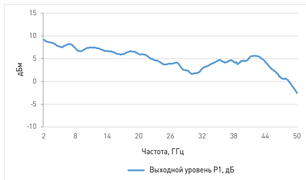
Рисунок 3-19 Keysight U7227F, зависимость выходного уровня P1 от частоты (типовая)
