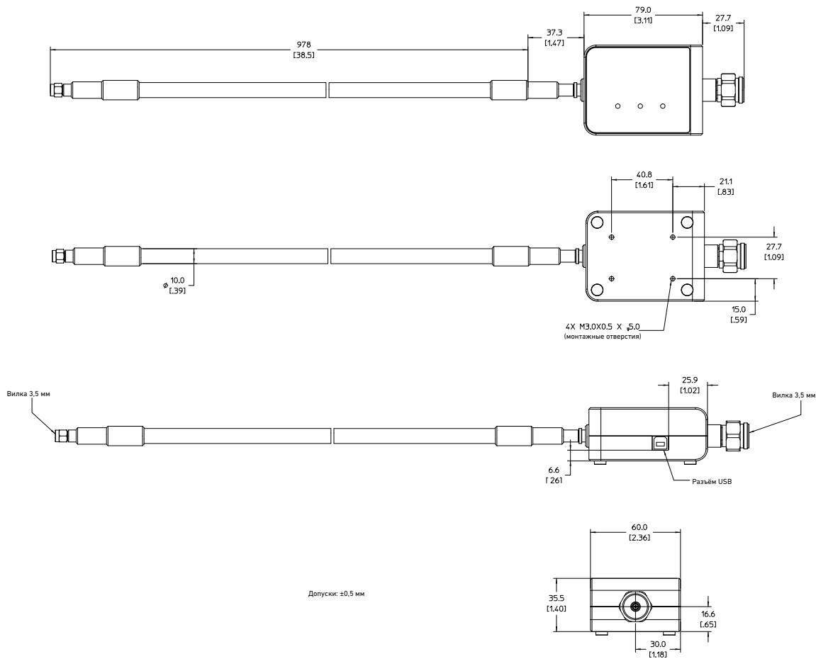
Рисунок 3-22 Размеры U7227A/C
