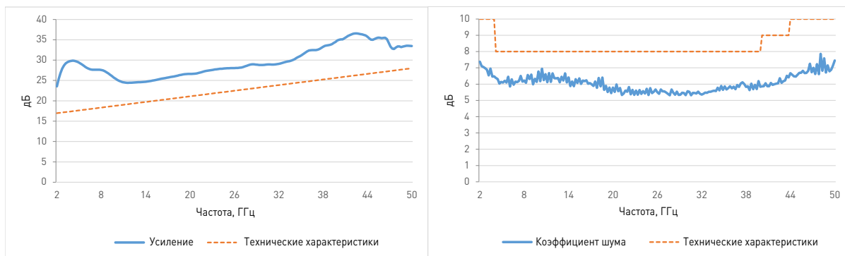
Рисунок 3-15 Keysight U7227F, зависимость усиления от частоты (типová)
