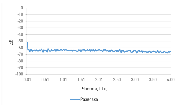
Рисунок 3-6 Keysight U7227A, зависимость развязки от частоты (типичная)
