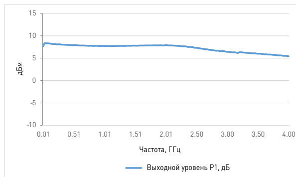
Рисунок 3-5 Keysight U7227A, зависимость выходного уровня P1 от частоты (типичная)
