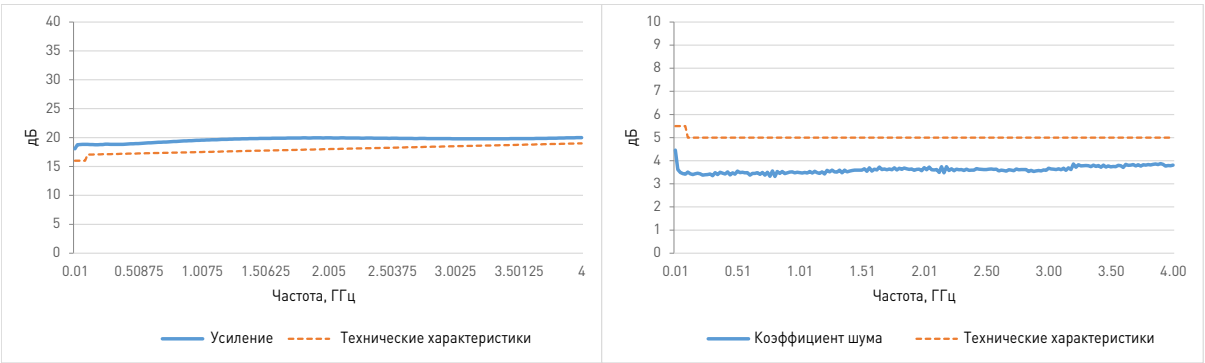
Рисунок 3-1 Keysight U7227A, зависимость усиления от частоты (типичная)
