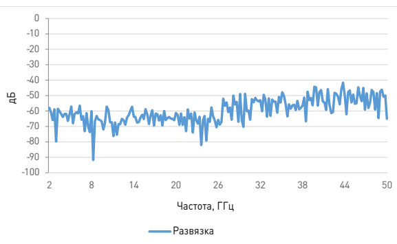
Рисунок 3-20 Keysight U7227F, зависимость развязки от частоты (типовая)
