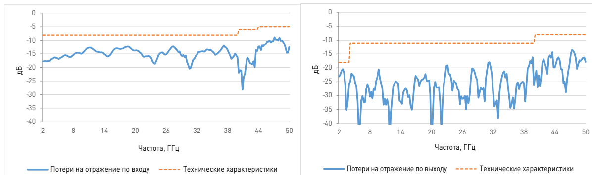
Рисунок 3-17 Keysight U7227F, зависимость потерь на отражение по входу от частоты (типová)
