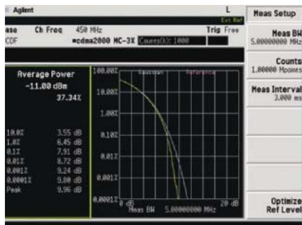
Измерение дополняющей интегральной функции распределения сигнала cdma2000 с четырьмя несущими
