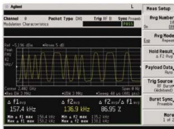
Характеристика модуляции
