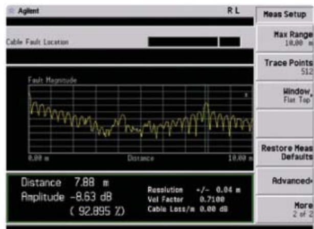
Вычисление расстояния до места повреждения в кабеле
