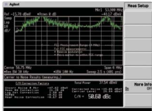
Измерение отношения сигнал/шум
